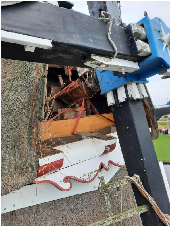
De oude windpeluw is hier weggehaald en dus staat het wiekenkruis op een krik en vastgezet met de nodige spanbanden.
